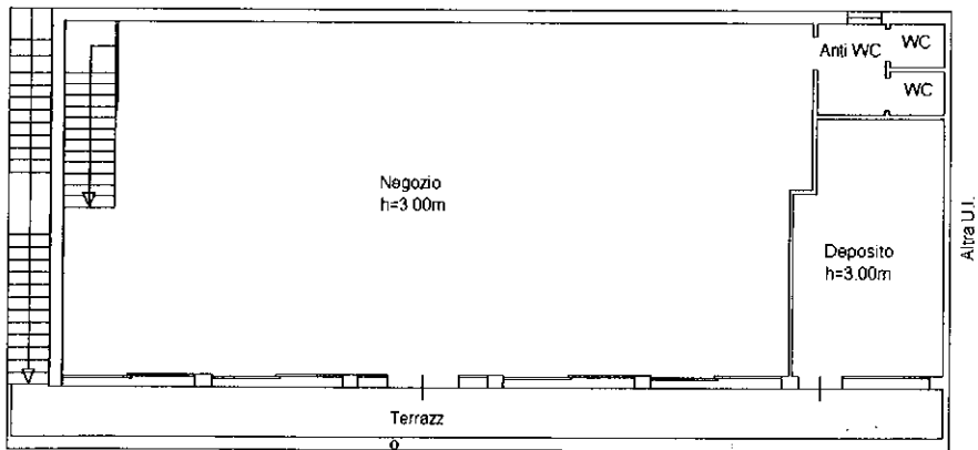
PIANO PRIMO h=2.70m
