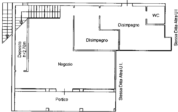
PIANO TERRA h=3.00m
